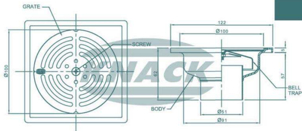
FLOOR DRAIN MODEL : 400 S (สำหรับท่อ PVC ขนาด 2"-4")
