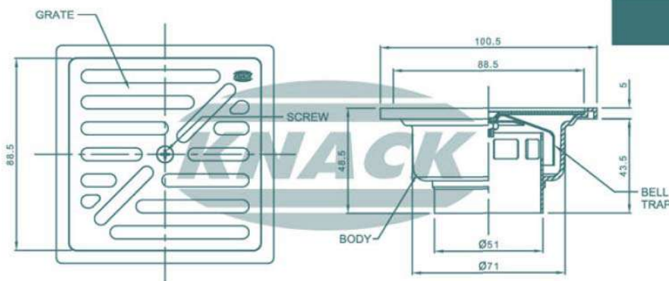
FLOOR DRAIN MODEL : 300 Z (สำหรับ PVC ขนาด 2"-3")
