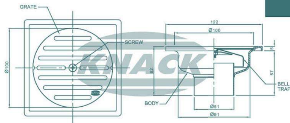
FLOOR DRAIN MODEL : 402 S (สำหรับท่อ PVC ขนาด 2"-4")
