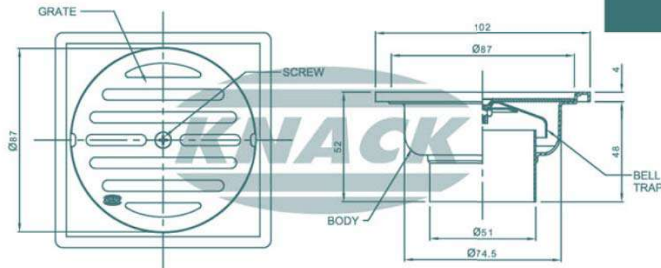
FLOOR DRAIN MODEL : 312 S (สำหรับ PVC ขนาด 2"-3")
