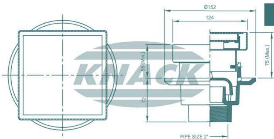
FLOOR DRAIN (หน้าตะแกรงสแตนเลส) แบบดักกลับ MODEL : 227 B (ขนาด 2")
