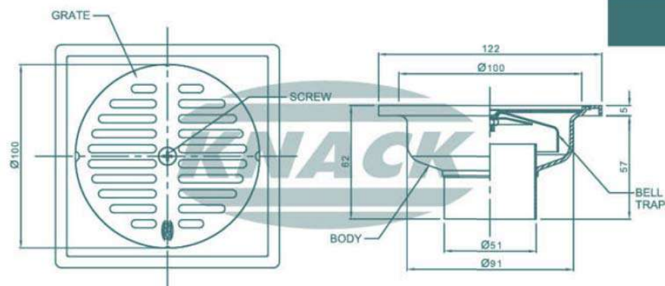
FLOOR DRAIN MODEL : 401 S (สำหรับท่อ PVC ขนาด 2"-4")
