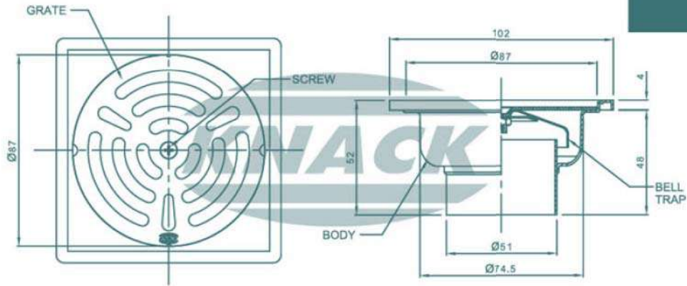
FLOOR DRAIN MODEL : 303 S (สำหรับ PVC ขนาด 2"-3")
