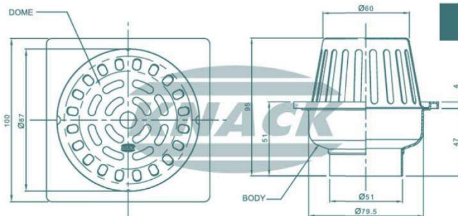
ROOF DRAIN MODEL : 320 S (สำหรับ PVC ขนาด 2"-3")
